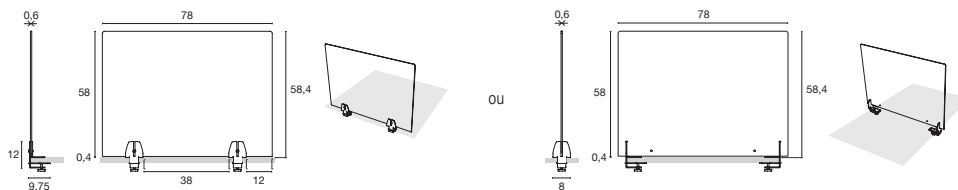
③ Panneaux périphérique ou intermédiaire avec débord de chaque côté (Inclus lot de pincés à double usage)
