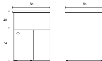
Modules hauts d'angle
