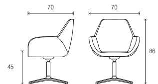
Piètement central 4 branches (1)
