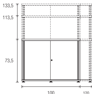
Bibliothèque avec 2 portes battantes
