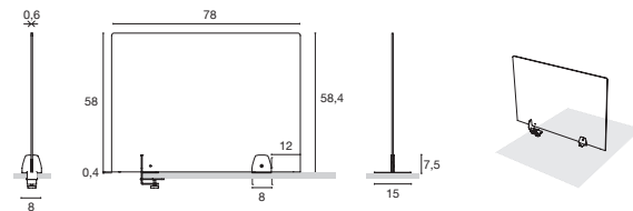
③ Panneaux périphérique ou intermédiaire avec débord de chaque côté (Inclus lot de pincés à double usage)
