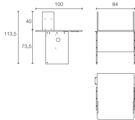
Module PMR* assis (intermédiaire)
