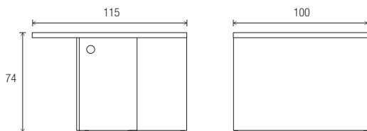
Module bas PMR***
