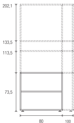
Bibliothèque sans portes
