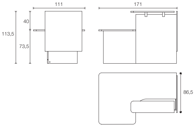
Module PMR* assis/debout (indépendant ou extrémité)
