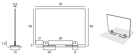
③ Panneaux périphérique ou intermédiaire avec débord de chaque côté (Inclus lot de pincés à double usage)
